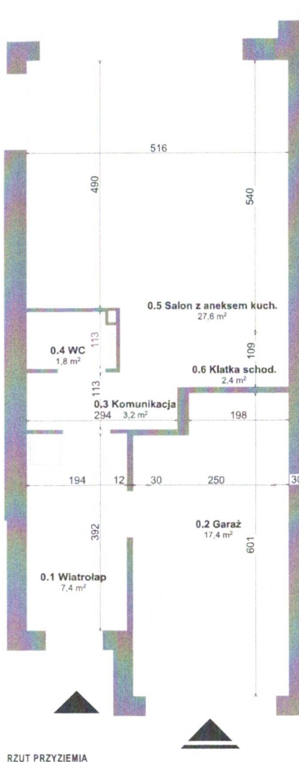
RZUT PRZYZIEMIA
