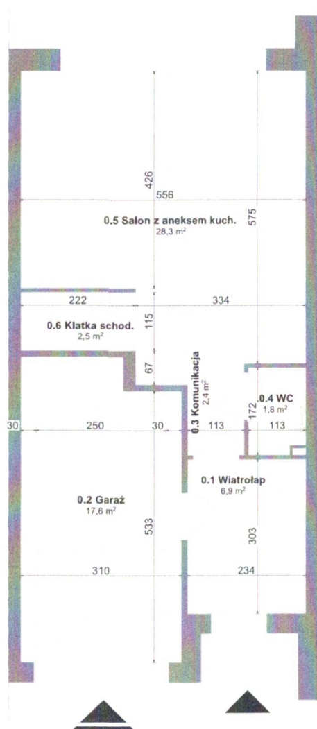
RZUT PRZYZIEMIA
