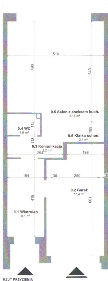
RZUT PRZYZIEMIA
