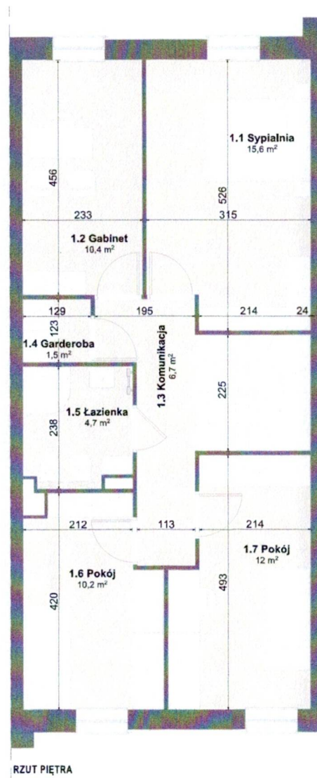
RZUT PIĘTRA
