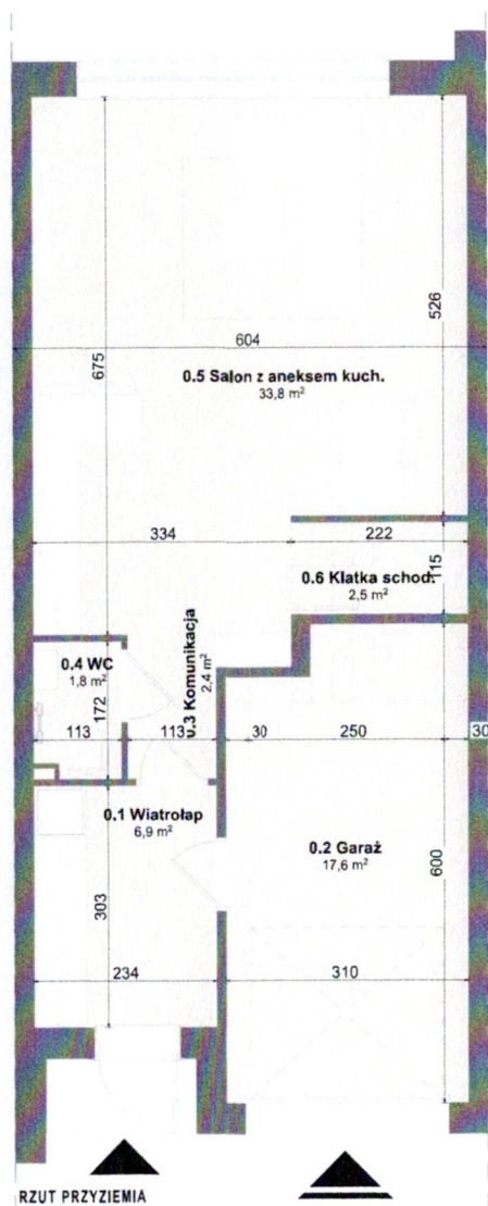
RZUT PRZYZIEMIA
