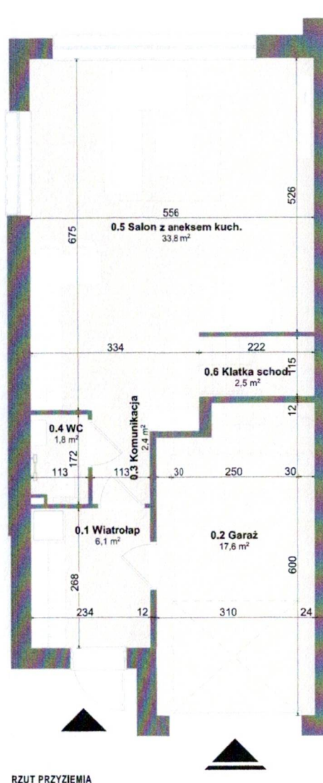
RZUT PRZYZIEMIA
